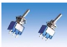
Interrupteur à bascule ON-OFF-ON 3pin 5A 250VAC /// YB-103
