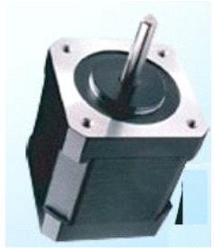
18303653 Moteur pas a pas 24V 6wire 1.2A 180° /// 42HZ48612N
