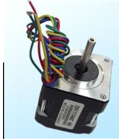
18303654 Moteur pas a pas 24V 4wire 1.2A 180° 39mm /// 39HZ3812
