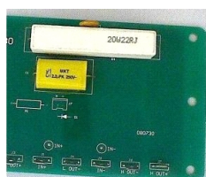
PCB filter pour RSX 15P80 /// RSX15P80
